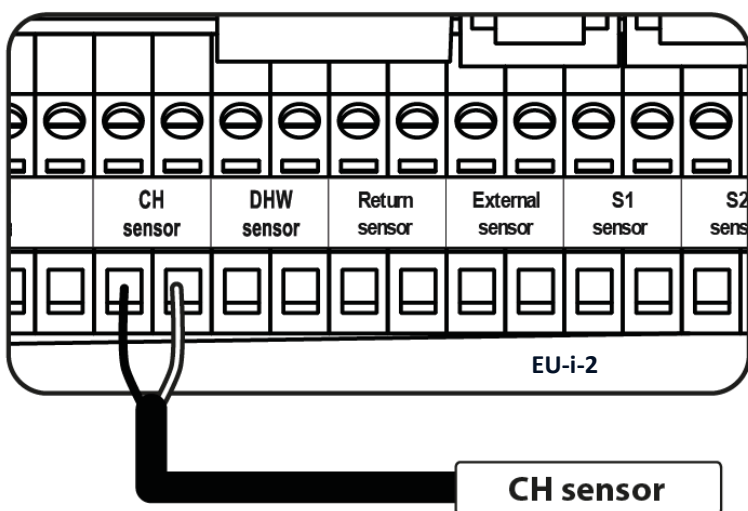
KF-szenzor csatlakoztatása
