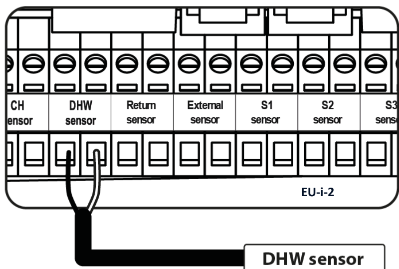
HMV-érzékelő csatlakoztatása
